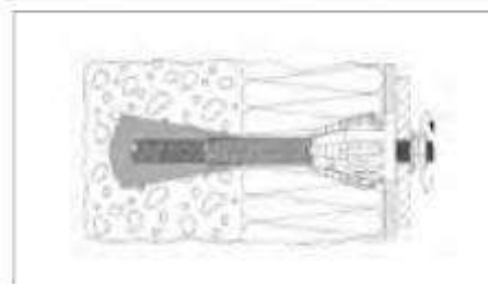
5 Fissaggi speciali su pannello isolante minerale TERMAX
