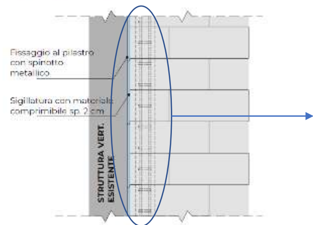
BLOCCO FORATO per irrigidimenti verticali
